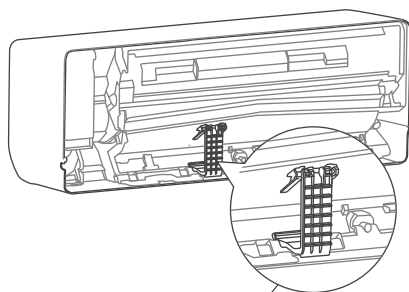
Runkotukipidike laitteen takana
