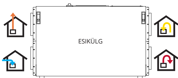
LIITMIKE PAIKNEMISE NÄIDE (külma õhu kanalid asuvad vasakul)
