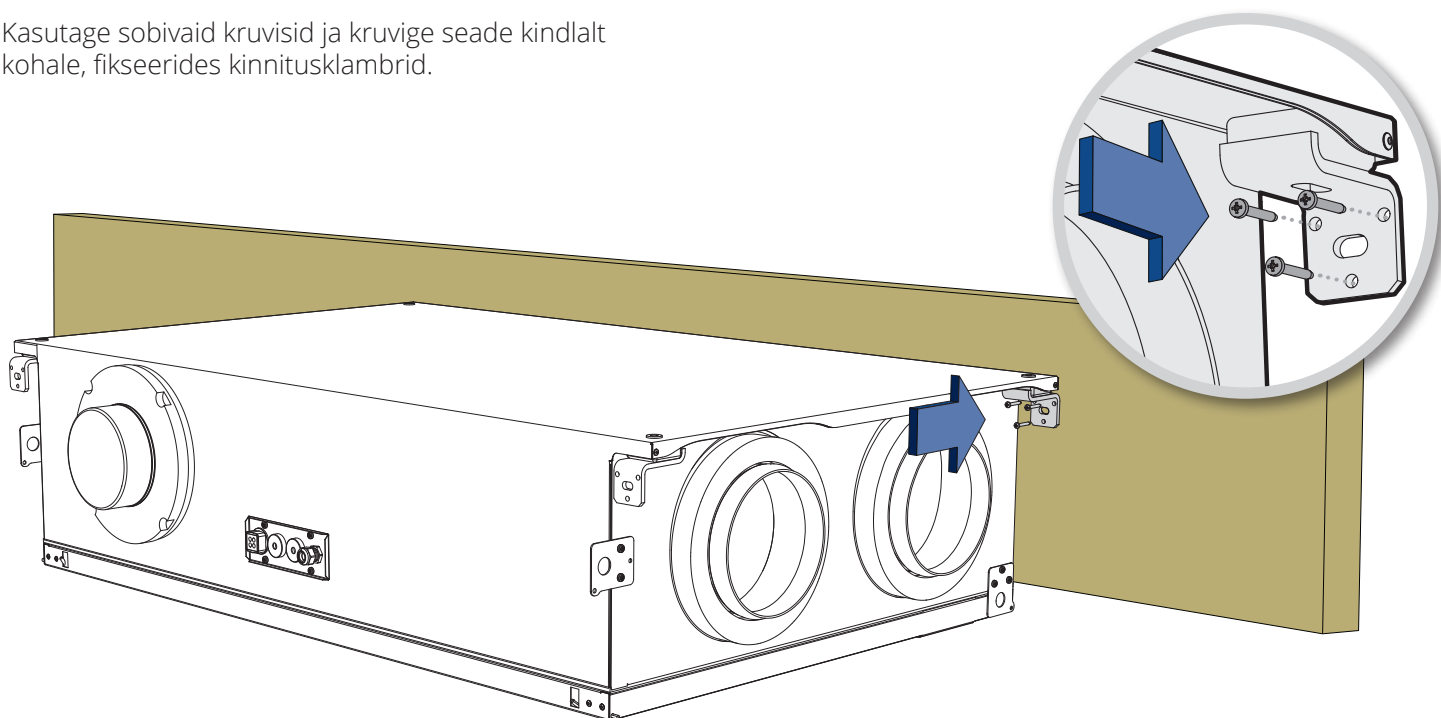
Joonis 10. Külgkinnitus
