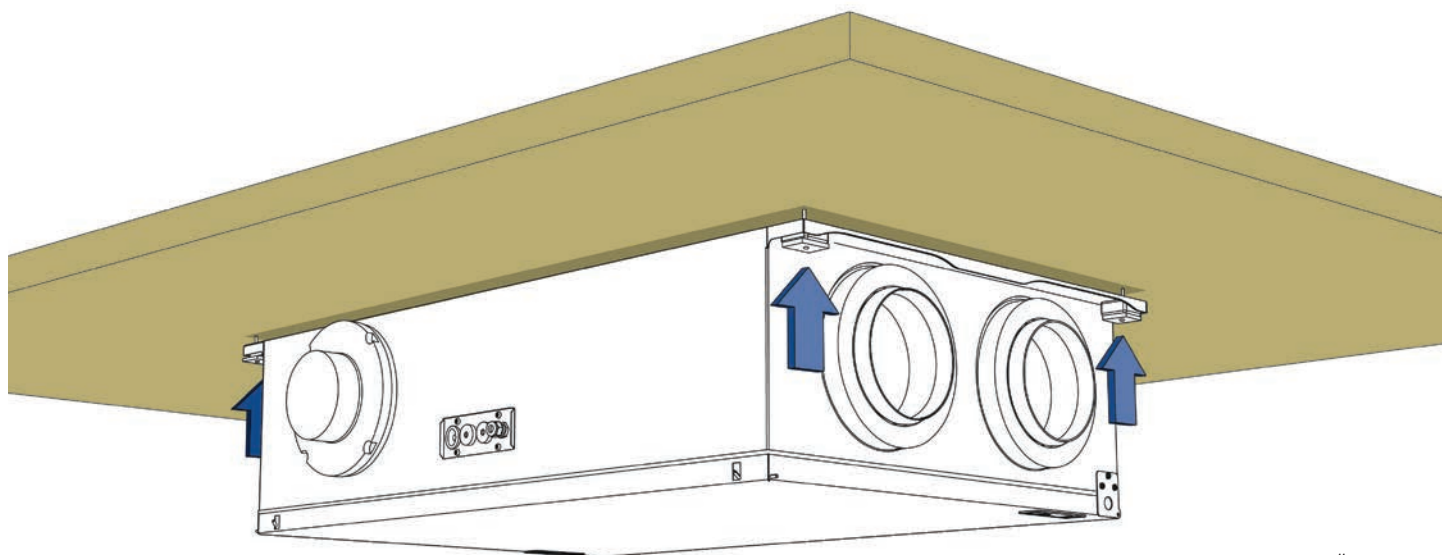
Joonis 8. Ülakinnitus
