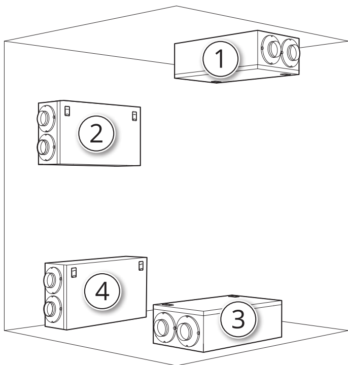
Joonis 2. Paigaldusvõimalused
